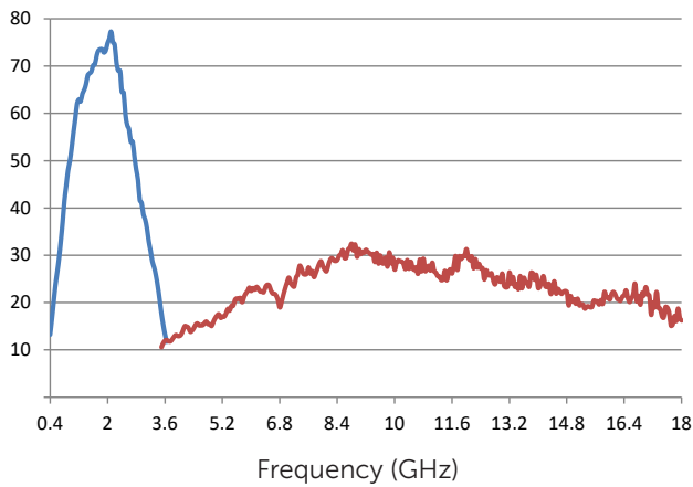
VSWR Lo/Hi
