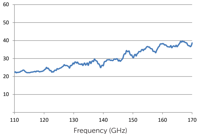
VSWR
