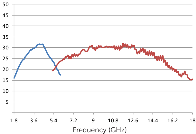
VSWR Lo/Hi
